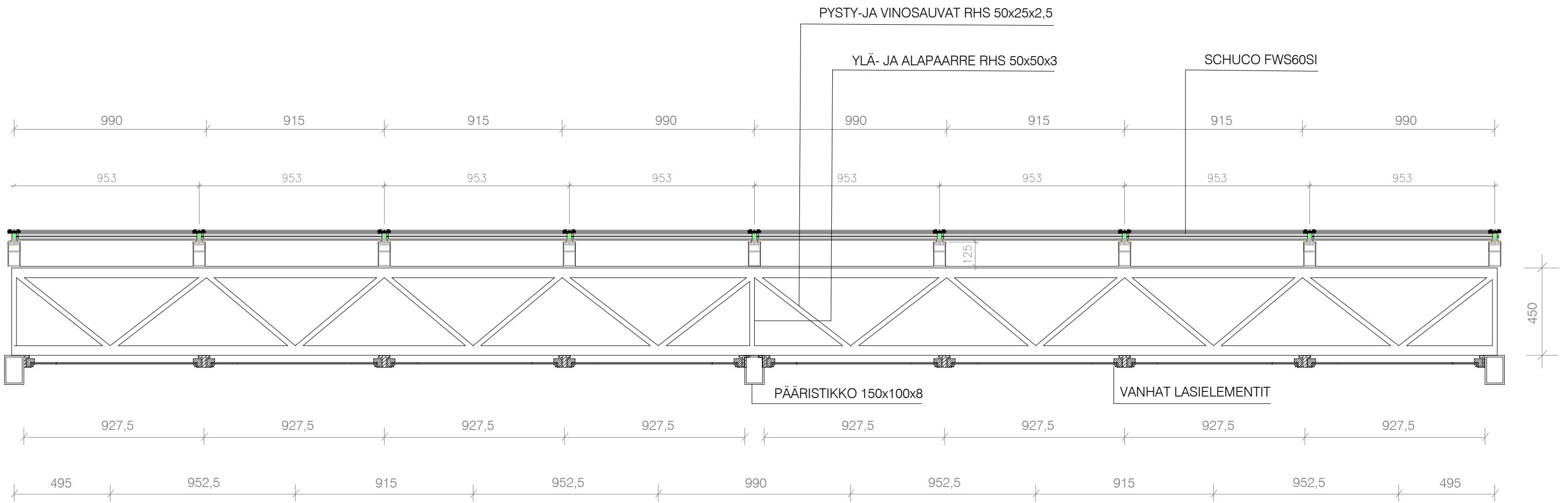
Leikkaus B-B, 1:20 (uusi ikkuna)
